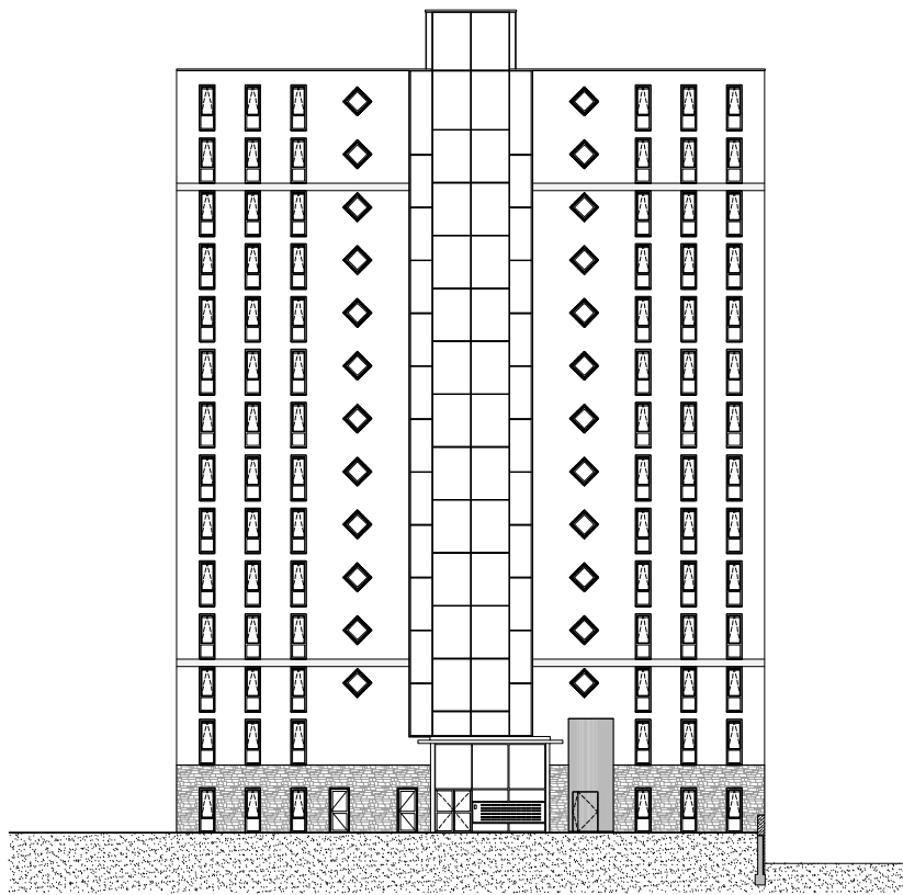
oostgevel
