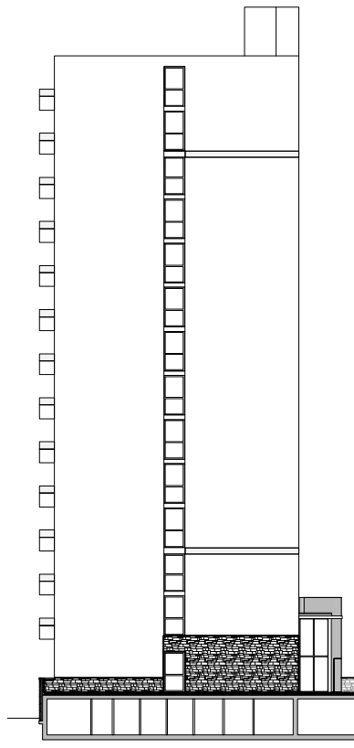
zuidgevel
