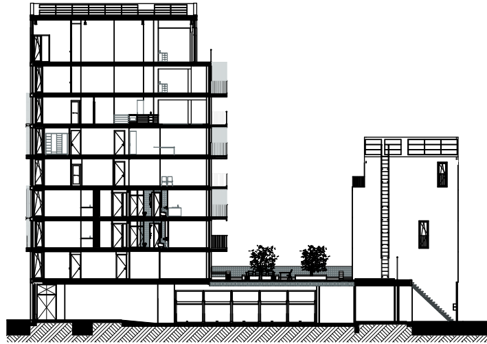
Doorsnede B
