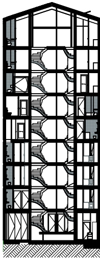
Doorsnede A
