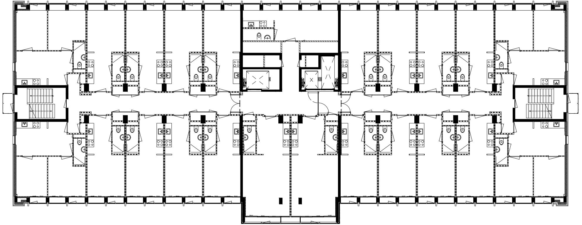
standaard plattegrond (verdieping 2 t/m10) 1:200
