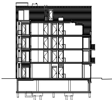
Dwarsdoorsnede parkeren
