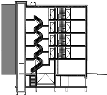
Dwarsdoorsnede inrit
