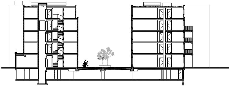
Doorsnede Wichersstraat
