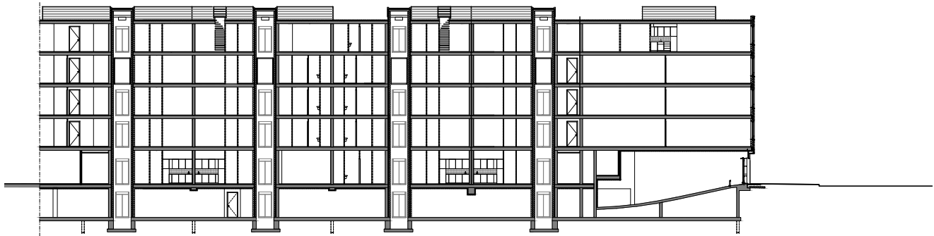
Dwarsdoorsnede inrit
