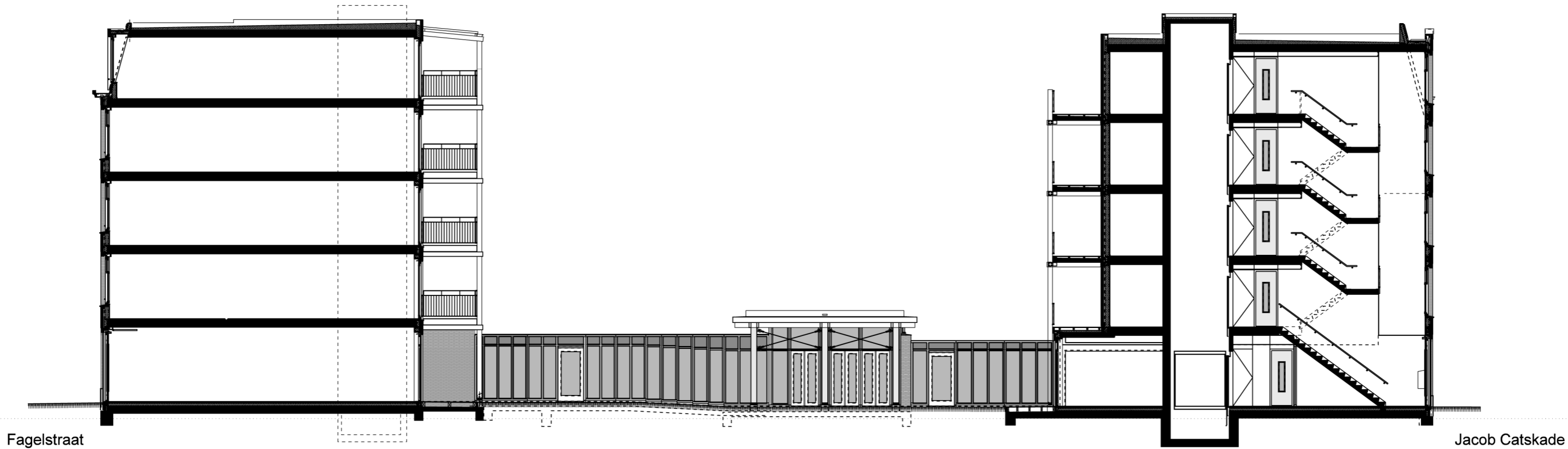
Doorsnede over binnenterrein
