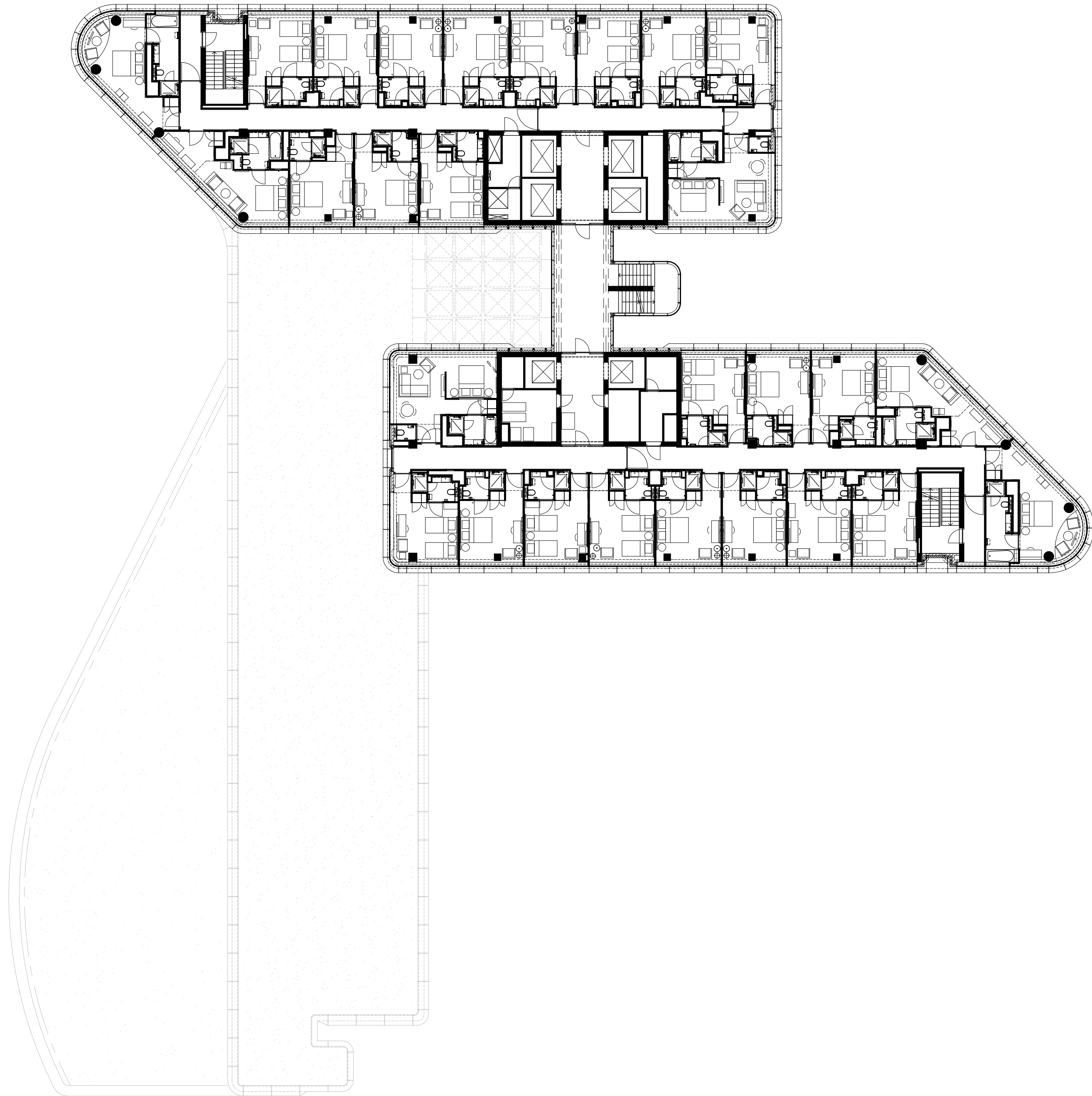
5e verdieping 1:200
