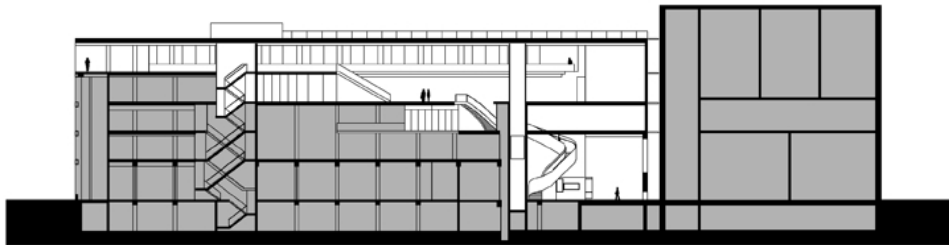
langsdoorsnede
