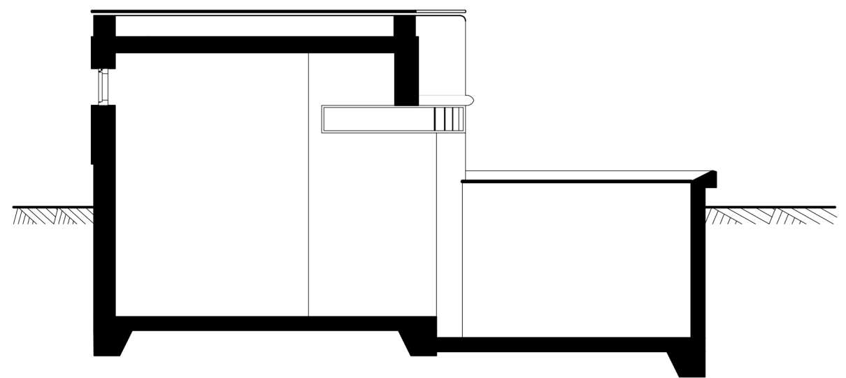
DOORSNEDE DAMES RETIRADE
