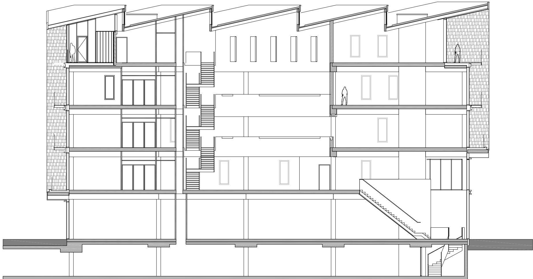
doorsnede 01
