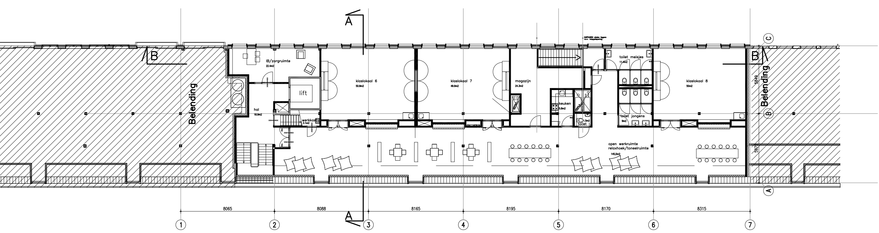
TWEDE VERDIEPING 462.1 m2 BVO
