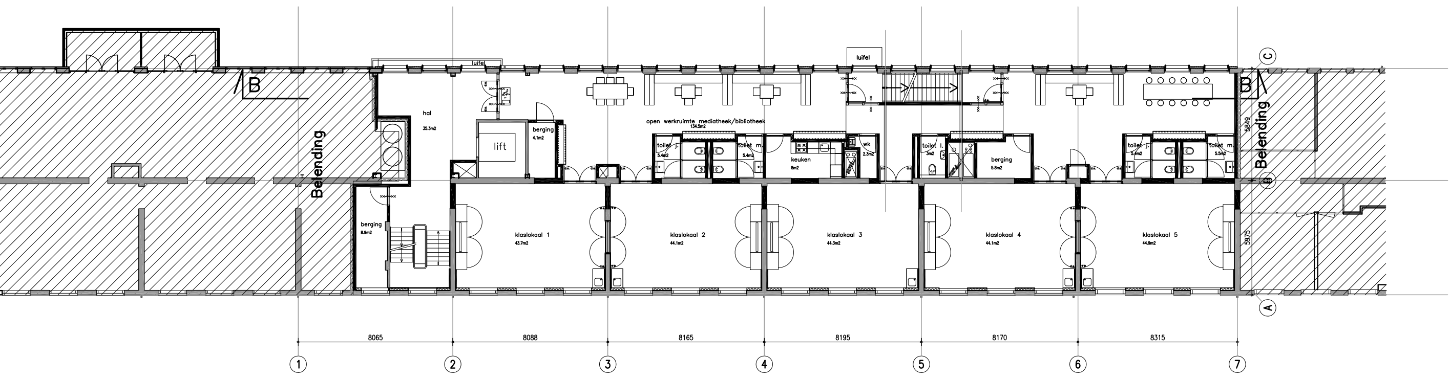
EERSTE VERDIEPING 540.1 m2 BVO
