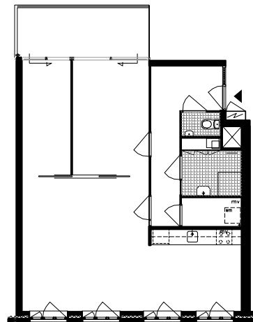
WoningtypeD3
