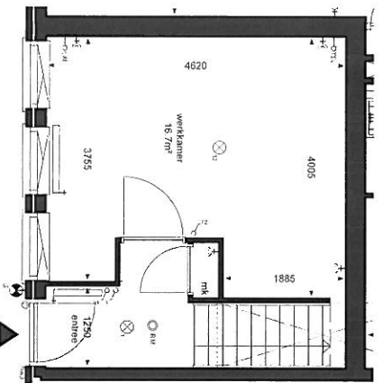
begane grond
