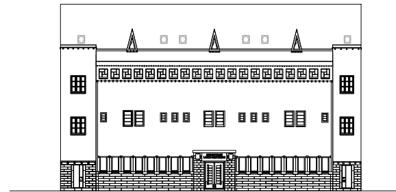
achtergevel NIEUW
