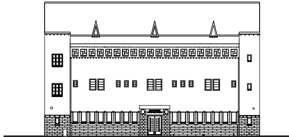
voorgevel BESTAAND
