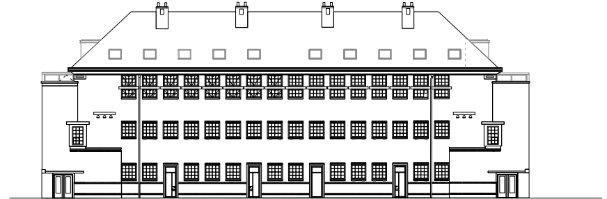
voorgevel NIEUW
