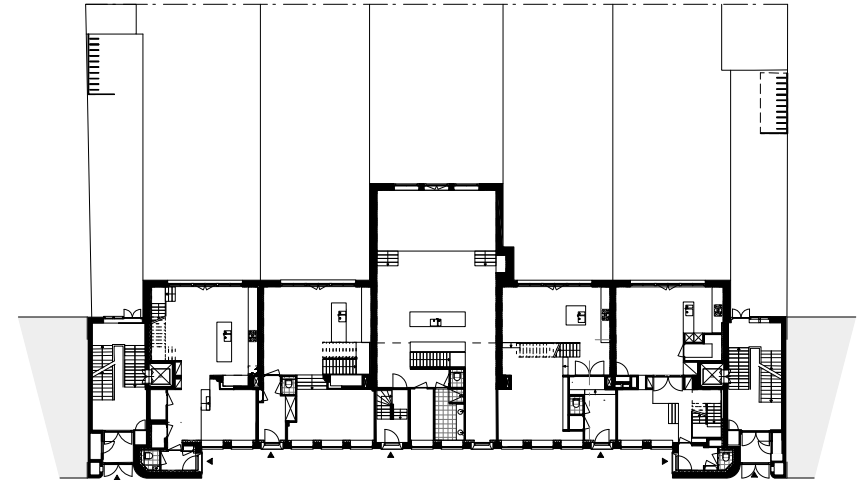
begane grond NIEUW
