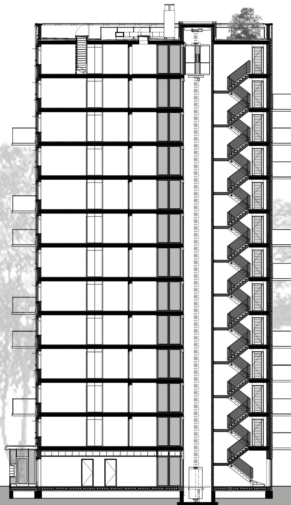
DOORSNEDE B-B
