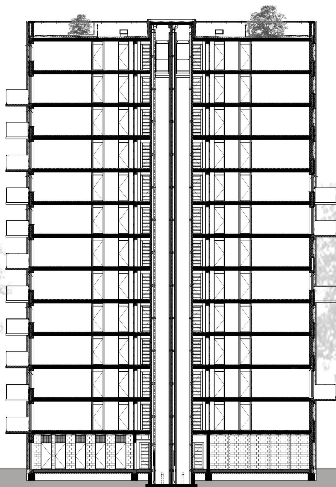
DOORSNEDE A-A
