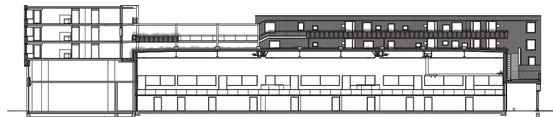
Doorsnede BB
