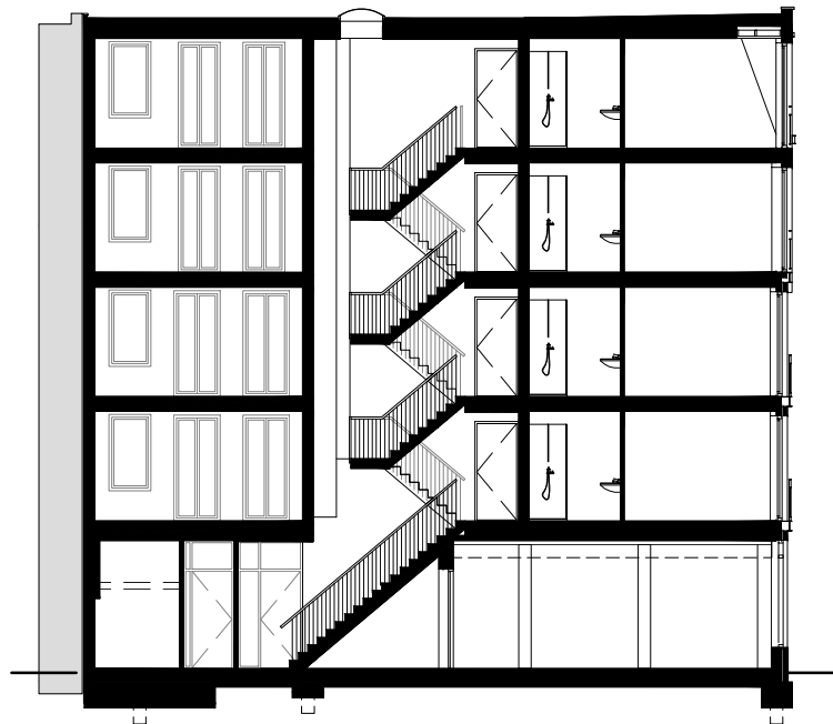
DOORSNEDE A
