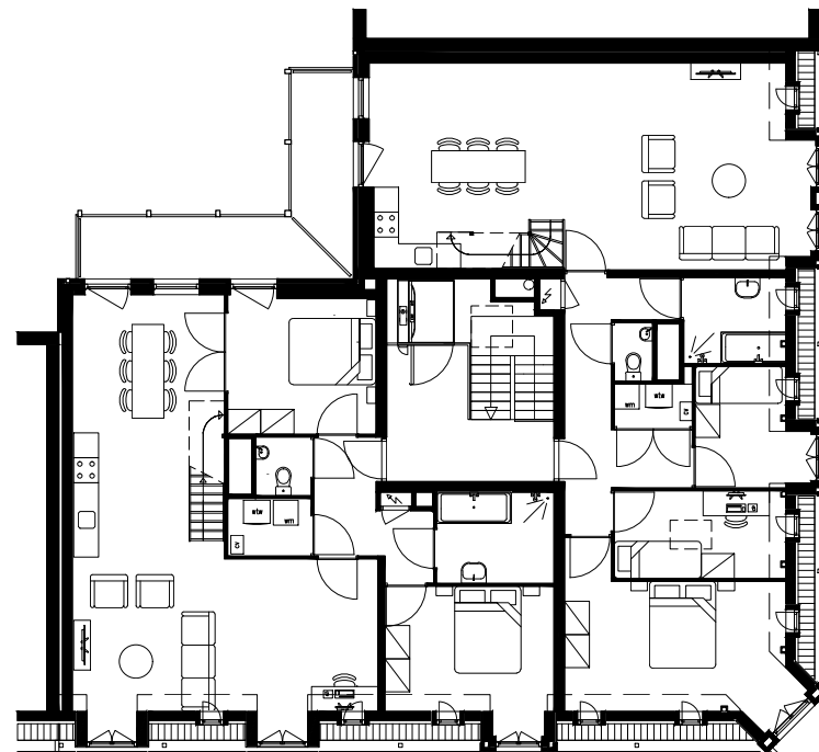
4E VERDIEPING
