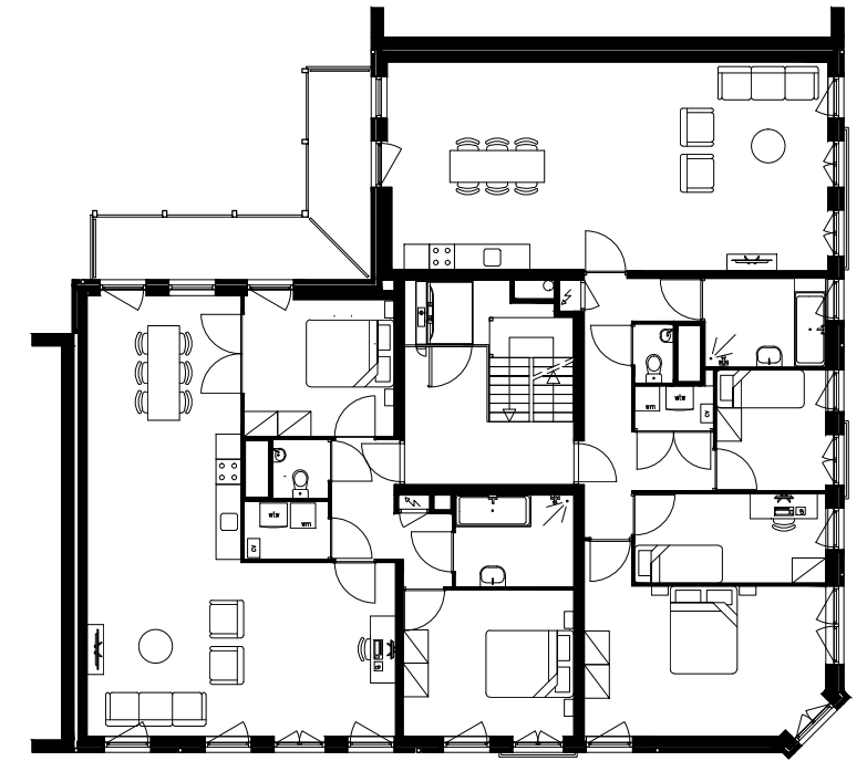
2E VERDIEPING
