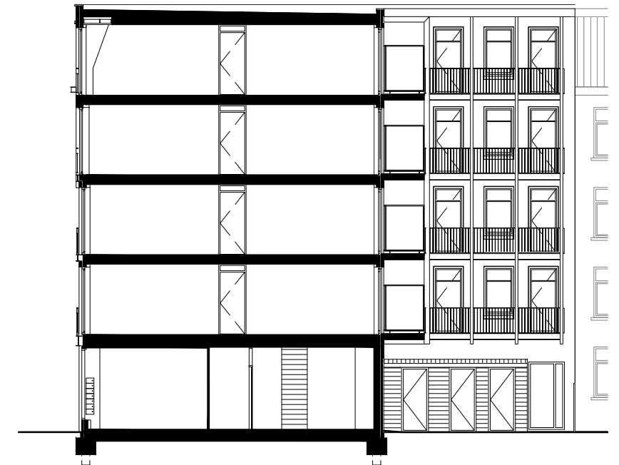
DOORSNEDE C
