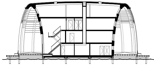
dwersdoorsnede B-B
